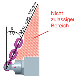
Abb. 4: Maximaler Neigungswinkel von 25° für WPP/WPPH-S/-B/-VIP
