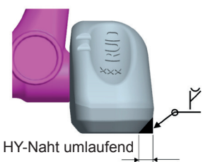
Abb. 3: HY-Naht
