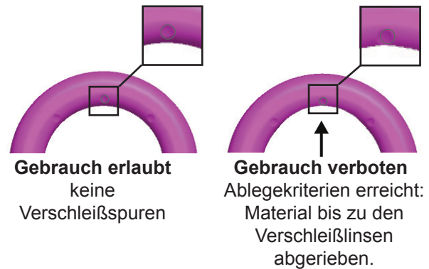
Abb. 1: Verschleißmarkierungen
