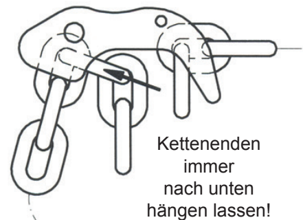
Bild 14: Montage / Anschluss Kranzkette
