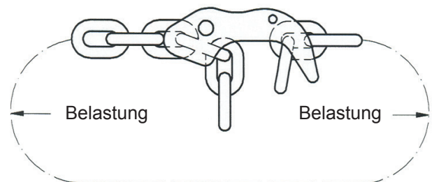
Bild 15: Montage / Anschluss Kranzkette
